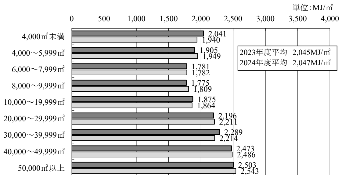
図 6 病院規模別にみた延床面積当たりエネルギー消費原単位（N=515、N=519）（再掲）
