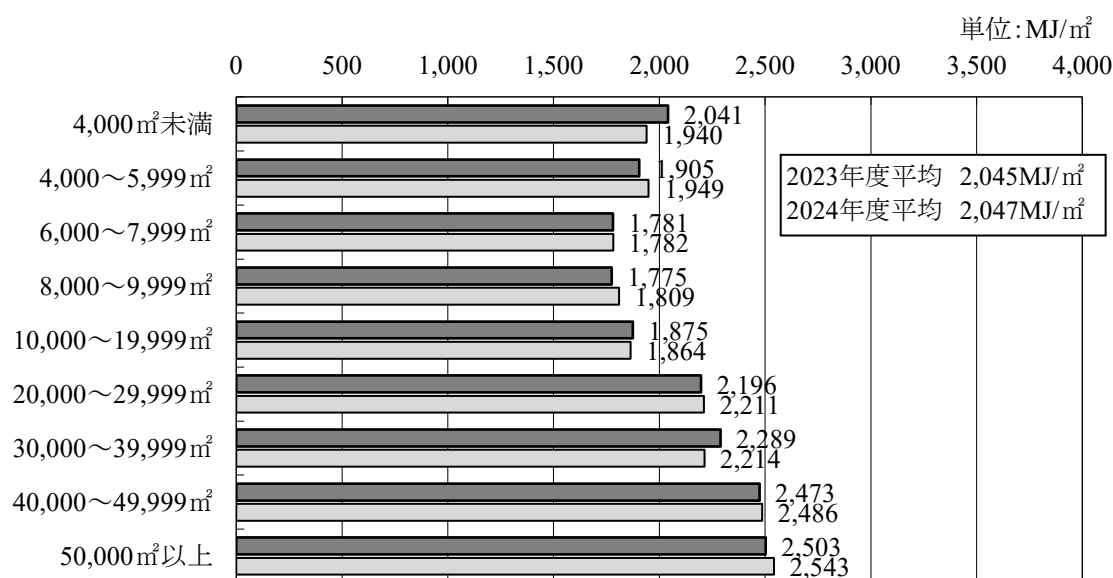
図 2 病院規模別にみた延床面積当たりエネルギー消費原単位 (N=539、N=541)
