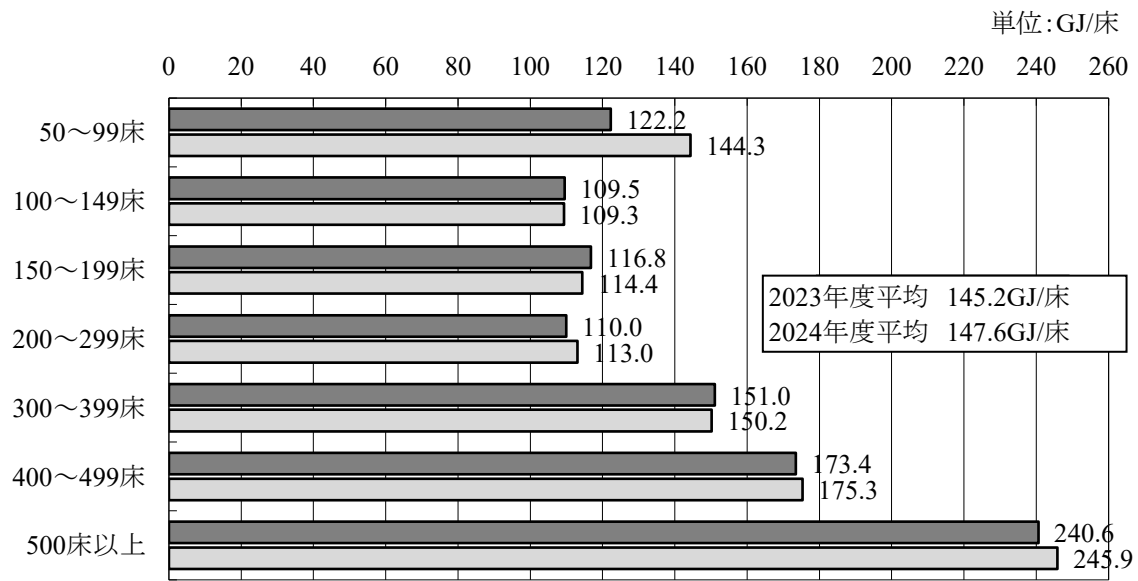
図 7 病院規模別にみた病床当たりエネルギー消費原単位 (N=515、N=519)
