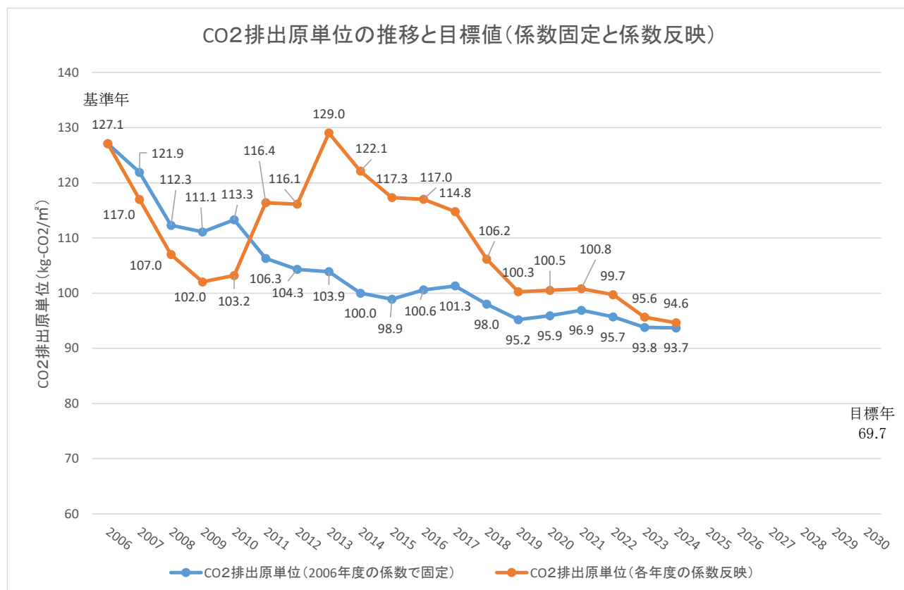
図 1 CO 2 排出原単位の推移と目標値
