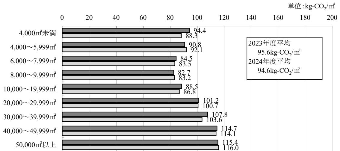
図 8 病院規模別にみた延床面積当たり CO 2 排出原単位 (N=515、N=519) (再掲)
