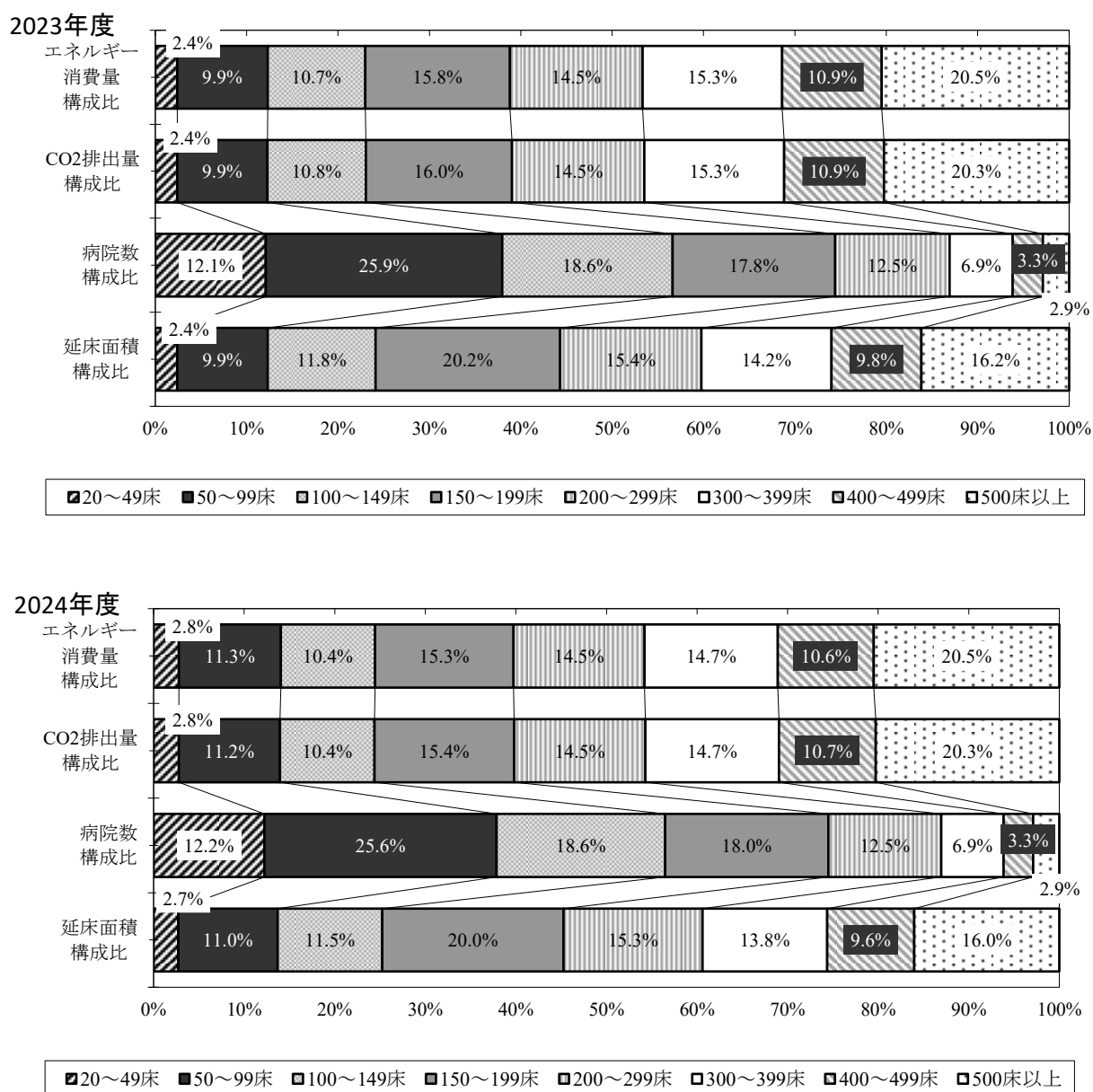
図 10 病床規模別にみたエネルギー消費量、CO 2 排出量の推計値の構成比（2023 年度、2024 年度）
