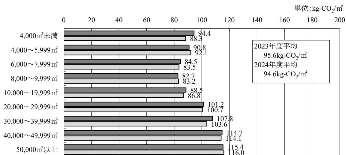
図 4 病院規模別にみた延床面積当たり CO 2 排出原単位 (N=515、N=519)
